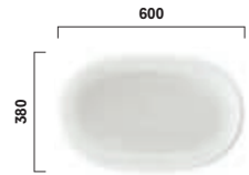
PJS05WEE#MW Aufsatzwaschtisch CE rund 600mm, ohne Hahnloch, mit Überlauf Vessel round 600mm, without tap hole, with overflow
