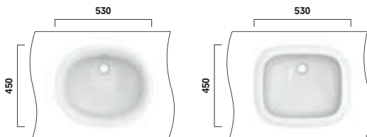
LW762Y Einbauwaschtisch rund 530mm, ohne Hahnloch, mit Überlauf Self-rim basin round 530mm, without tap hole, with overflow
