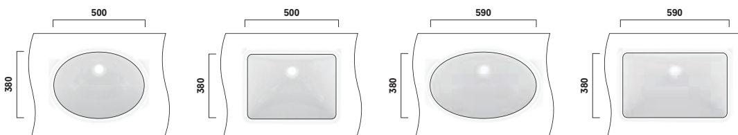
LW1505JUYW/F#W Unterbauwaschtisch WU, rund 500mm, ohne Hahnloch, mit Überlauf Undercounter basin WU round 500mm, without tap hole, with overflow
